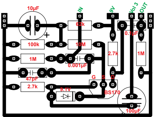
Schéma de montage AMZ Mosfet Booster
